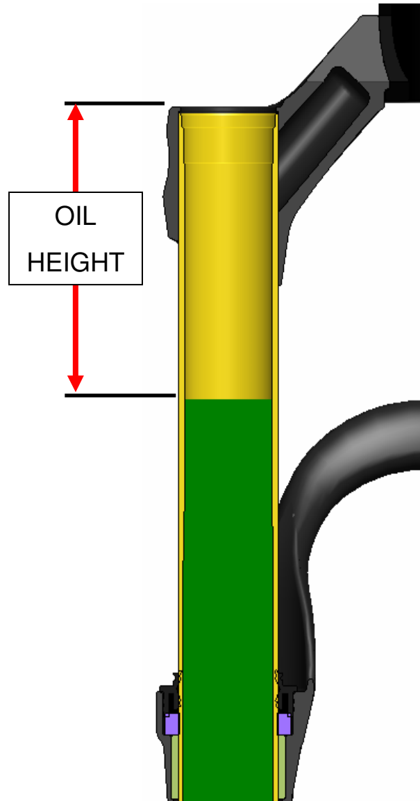
In-Leg Forks
