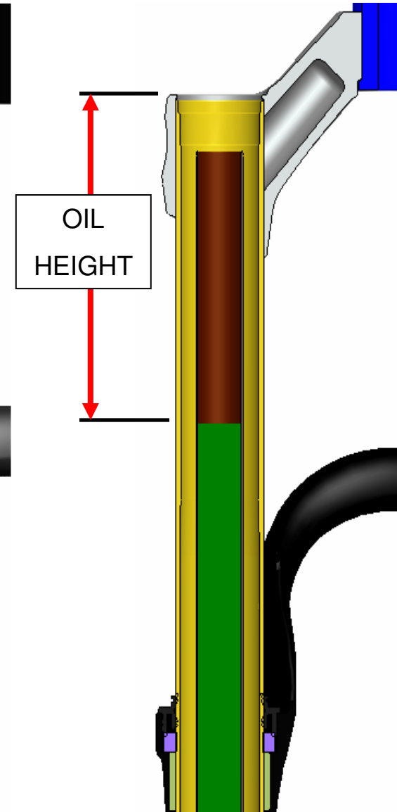
MRD Forks
